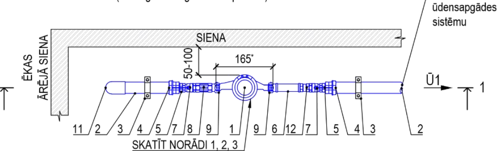
GRIEZUMS 2-2
