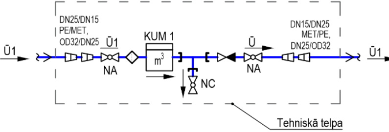
KUM1 MEZGLA SHĒMA
