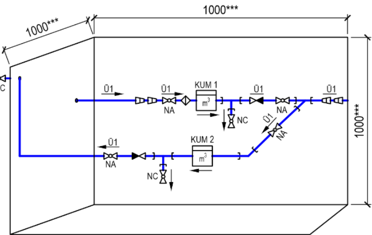
KUM1 UN KUM2 IZVIETOJUMA SHĒMA ĒKĀ
