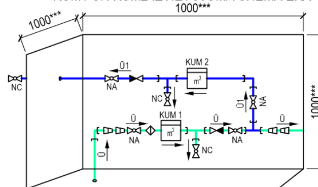
KUM1 UN KUM2 IZVIETOJUMA SHĒMA ĒKĀ
