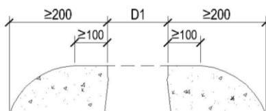
GRIEZUMS 3-3
