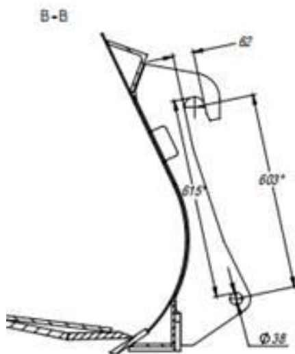
1.attēls. Ekskavatora-iekrāvēja JCB 3CX priekšējā kausa “ātrās sakabes” shematisks attēlojums
