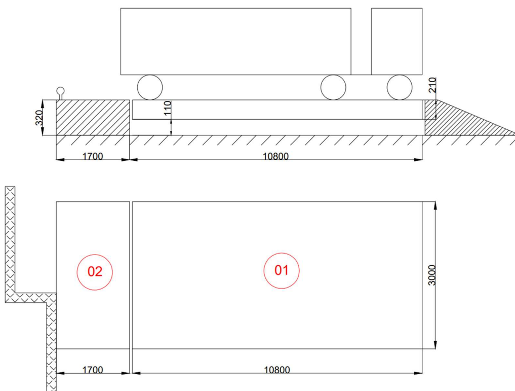
1.attēls Autosvaru konstrukcijas shēma
