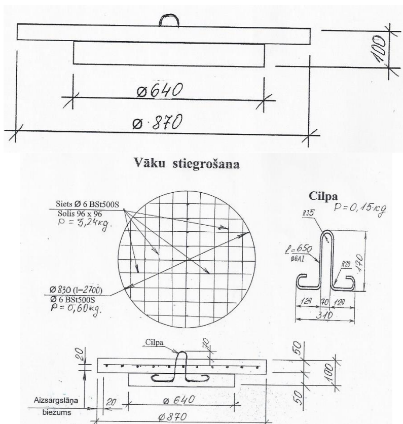
1.attēls Dzelzsbetona lūku vāks KLV-6
