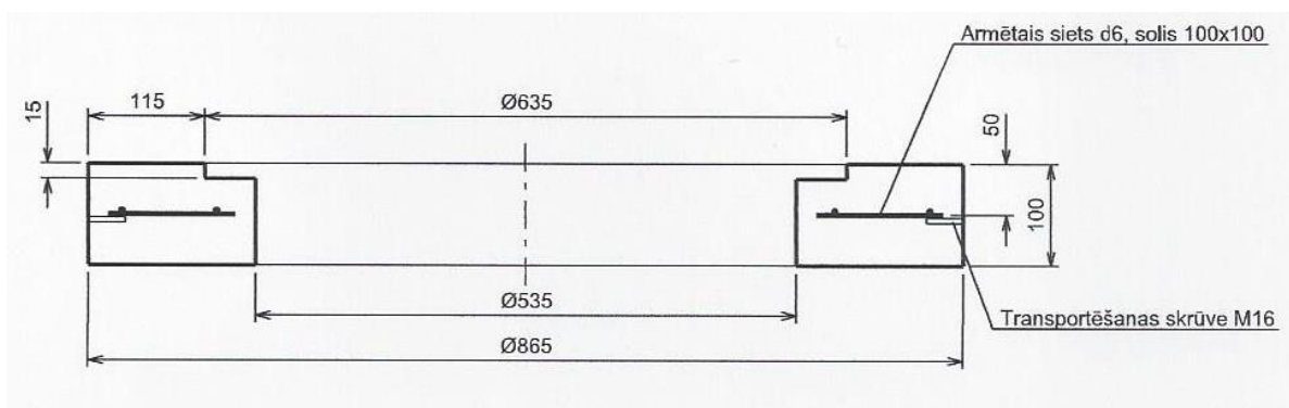
7.attēls Hidrantu lūkas aizsarggredzens: ārējais D-0,86-0,87m, iekšējais D-0,53-0,54m; H-0,10m
