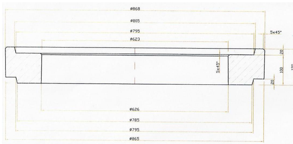
4.attēls Regulēšanas gredzens: ārējais D-0,86-0,87m, iekšējais D-0,62-0,63m; H-0,10m
