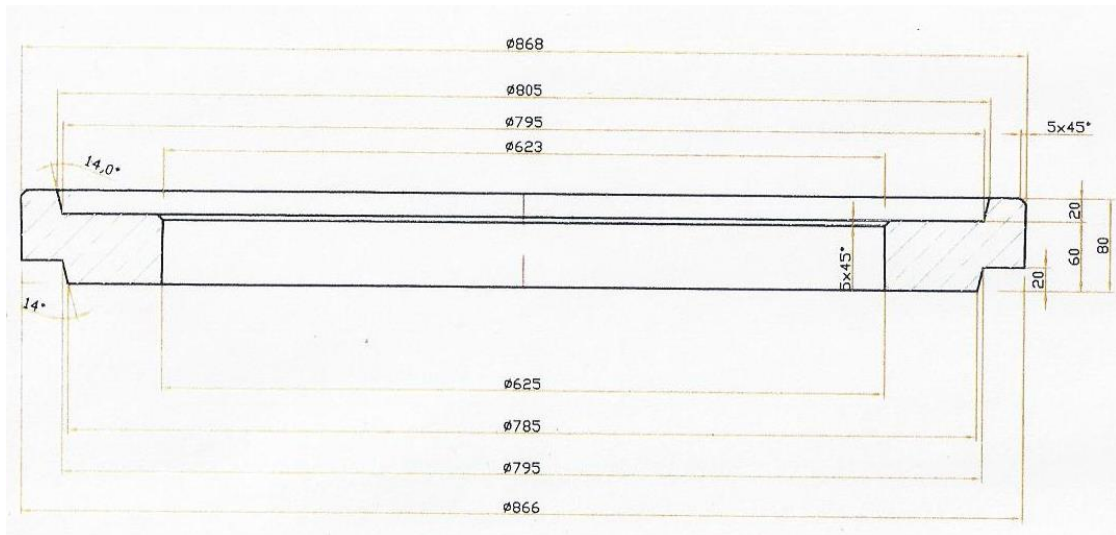
3.attēls Regulēšanas gredzens: ārējais D-0,86-0,87m, iekšējais D-0,62-0,63m; H-0,06m
