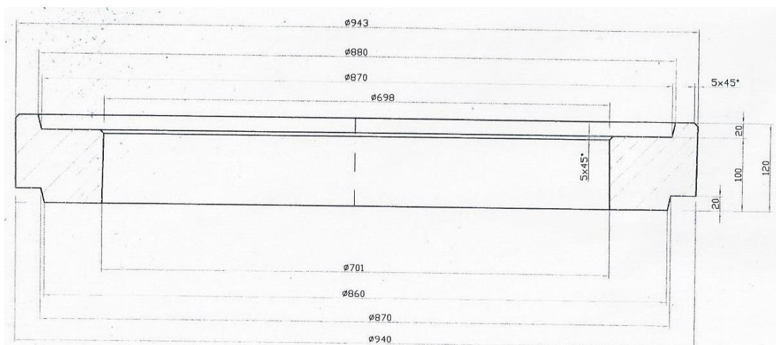
5.attēls Regulēšanas gredzens: ārējais D-0,94-0,95m, iekšējais D-0,69-0,70m; H-0,10m
