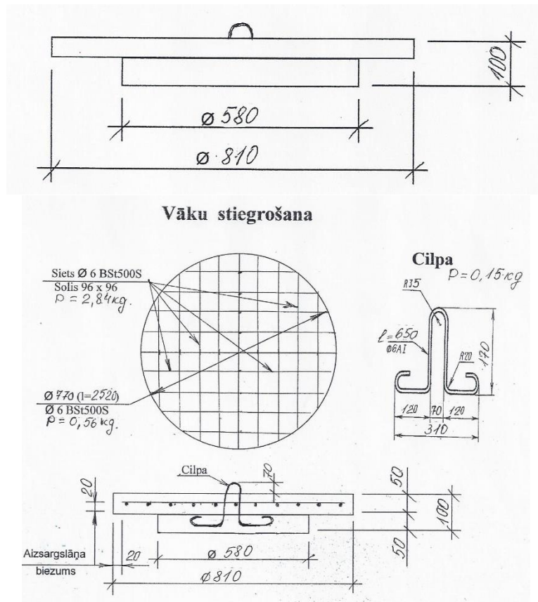
1.attēls Dzelzsbetona lūku vāks KLV-6
