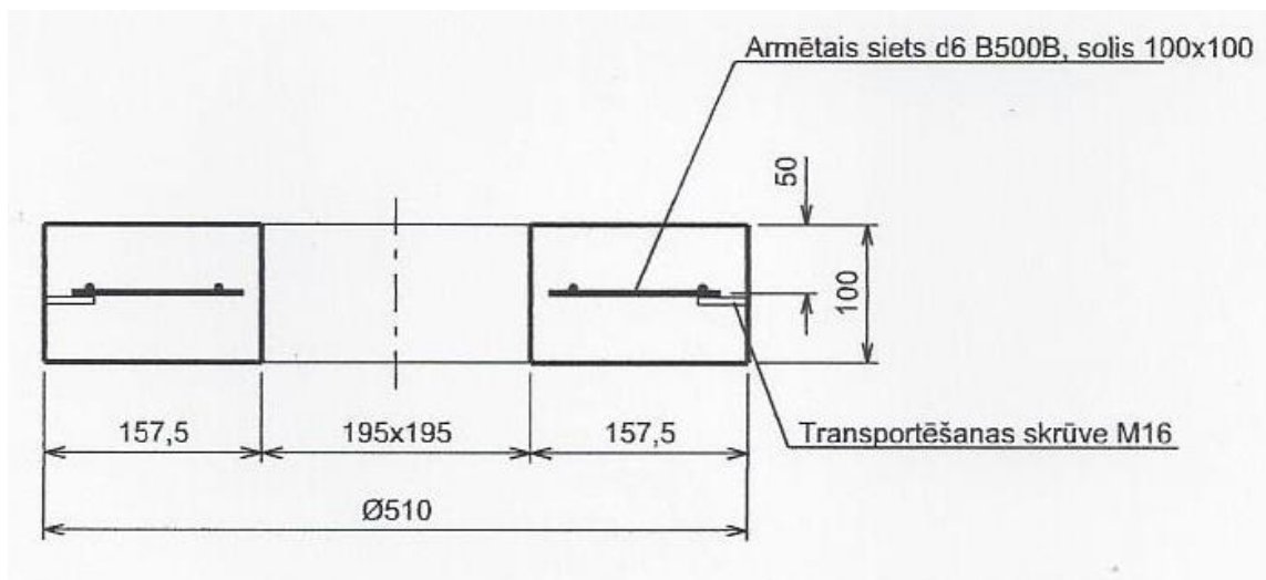
6.attēls Aizbīdņu kapes aizsarggredzens: ārējais D-0,50-0,51m, iekšējais D-0,195x0,195m; H-0,10m
